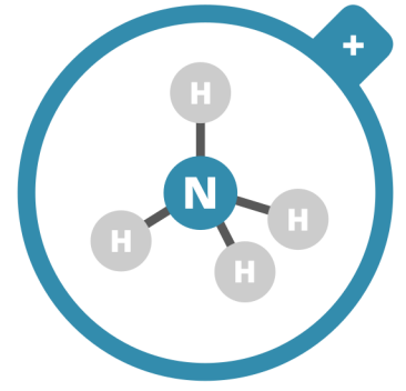
AMMONIUM
