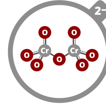
DICHROMATE
